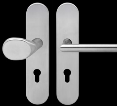
Schutzbeschlag ESG 675 Edelstahl matt SK2, ES1, RC3 und SKG***
