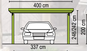
Modell „City-Carport 1“
